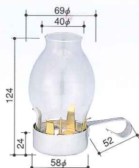
KB-1022 品名/持手付中 材質/アルミ 用途/ト一口火袋用
