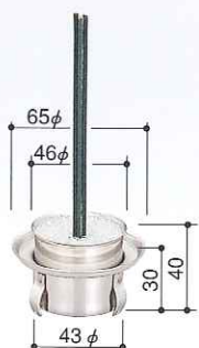
KB-3431 品名/1寸7分 材質/ステンレス・ 供養灰入り 用途/墓前
