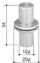
KB-3412 品名/12φ用回転軸 材質/ステンレス
