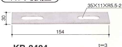
KB-3404 品名/平型・ボルト2本付 材質/ステンレス
