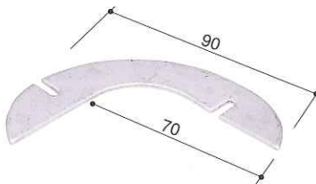
KB-3403 品名/コーナー 材質/ステンレス
