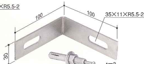
KB-3406 品名/L型B・ボルト2本付 材質/ステンレス
