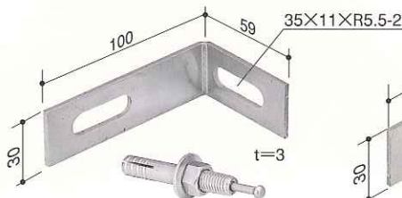
KB-3405 品名/L型A・ボルト2本付 材質/ステンレス
