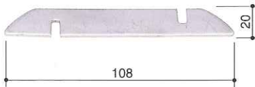
KB-3402 品名/一文字 材質/ステンレス
