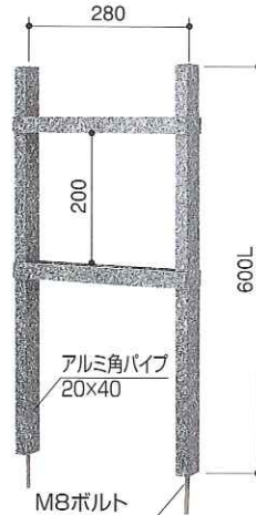
KB-6110-1 (ボルト付)
