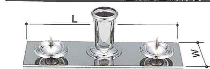
KB-2027 品名/線香・ローソク立セット(小) 寸法/ベースW60×L180 KB-2028 品名/線香・ローソク立セット(大) 寸法/ベースW113×L180
