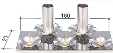
KB-2402 (特別製作品) 品名/屋形香立用線香・ローソク立セット
