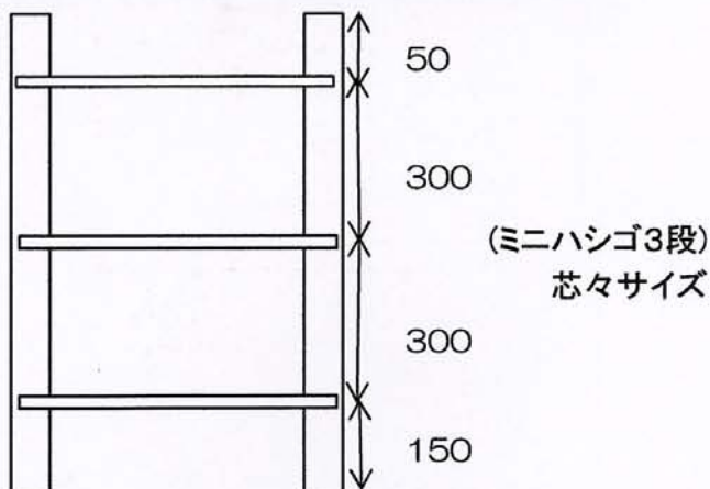
ミニハシゴ3段(ボルト・金具)付組立、柱800、スタンダード品
