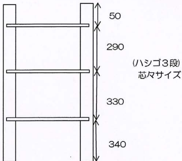
ハシゴ3段(ボルト・金具)付組立、柱1010、スタンダード品
